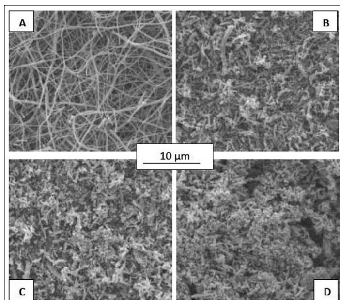
Fig. 5. SEM images of milled electrospun TiO 2 nanofibers (ET3). Milling time (A) 0 s, (B) 30 s, (C) 60 s, (D) 120 s.
